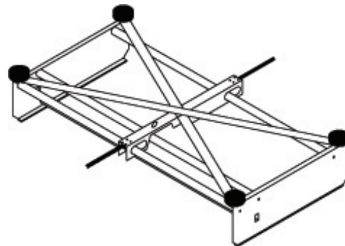
Kanalschieber unter Spaltenboden
