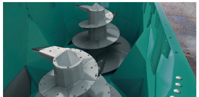
Rehusekoituksen valmistuksen apulaiset: hellävaraiset sekoitusruuvit ja leikkuuterät
